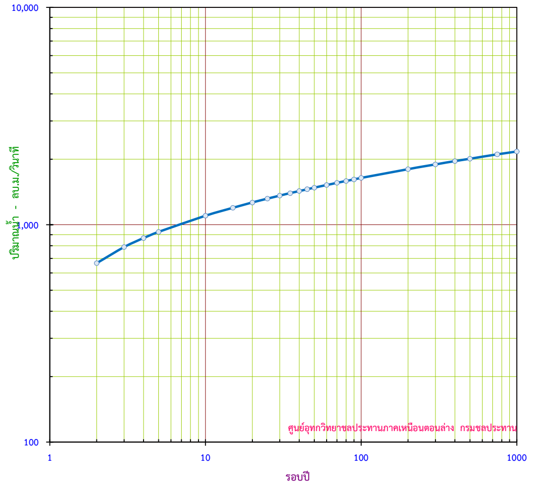
กราฟแสดง ปริมาณน้ำสูงสุดรายปี ขนาดรอบปีต่างๆ สถานี Y.33 อ.ศรีสำโรง จ.สุโขทัย
